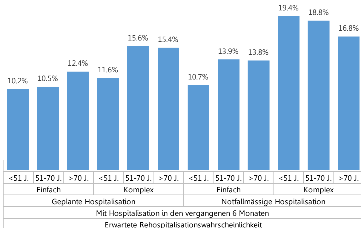
Abbildung 3: Adjustierungstabelle am Beispiel Schwere Infektion
