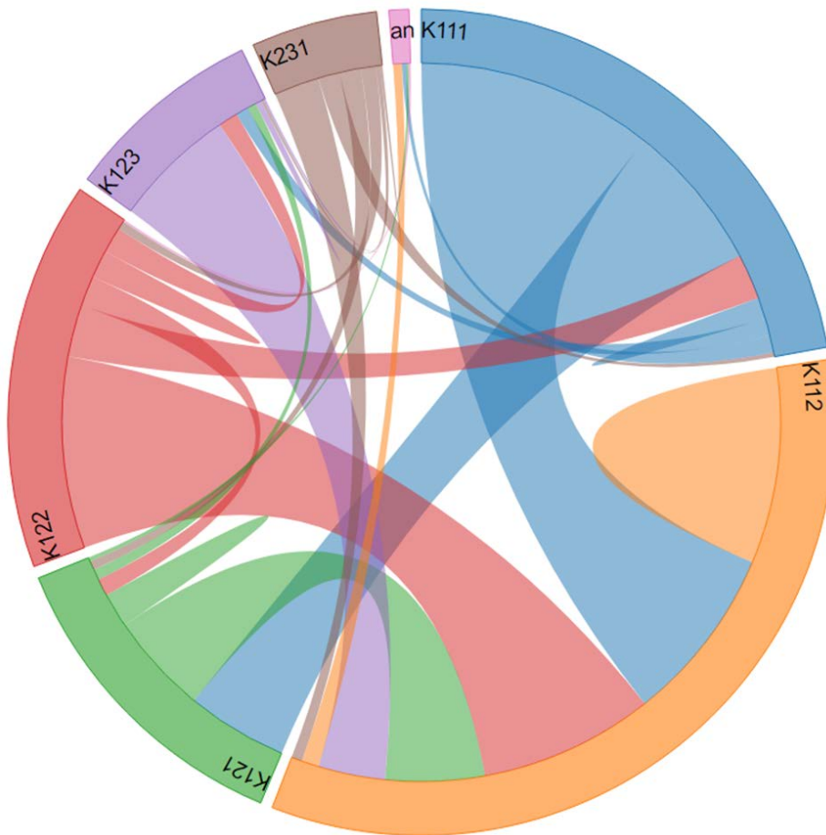
Abbildung 8: Chordgrafik Patientenströme
